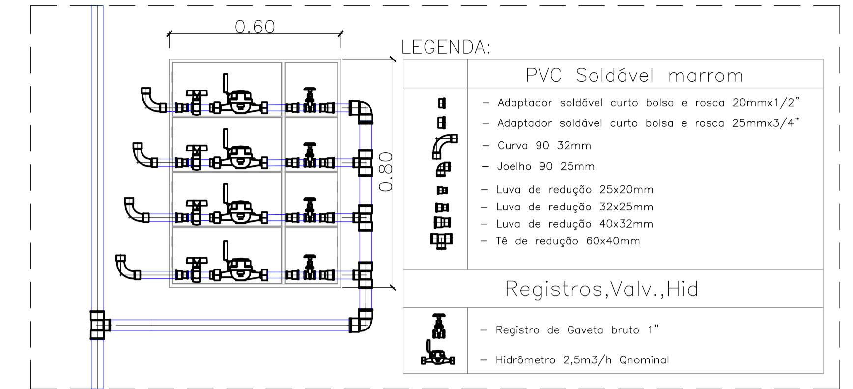
DETALHE - CAIXA DE HIDRÔMETRO SEM /ESC.
