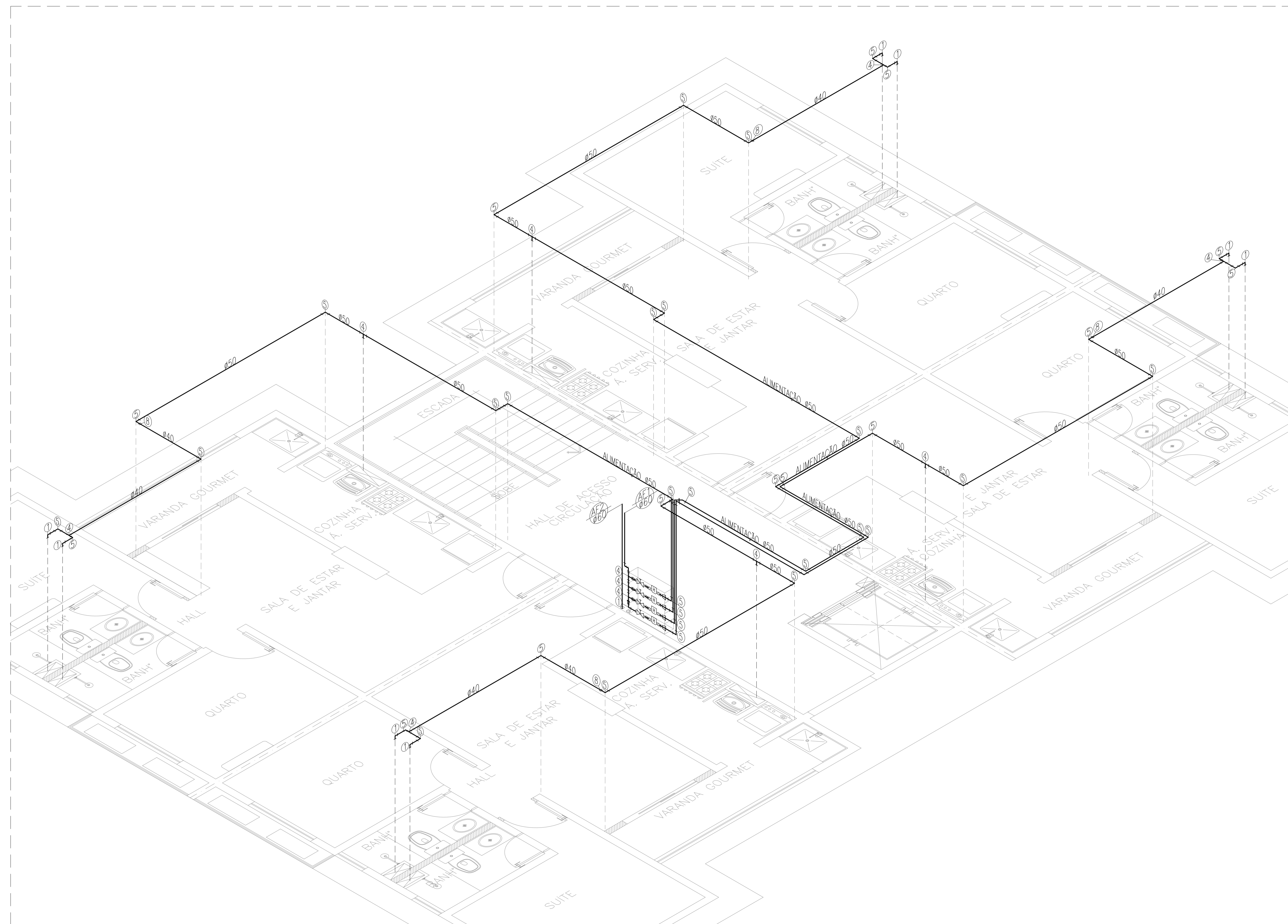
ISOMÉTRICO BLOCO TIPO B - 3º PAVIMENTO. ESC. 1/35
