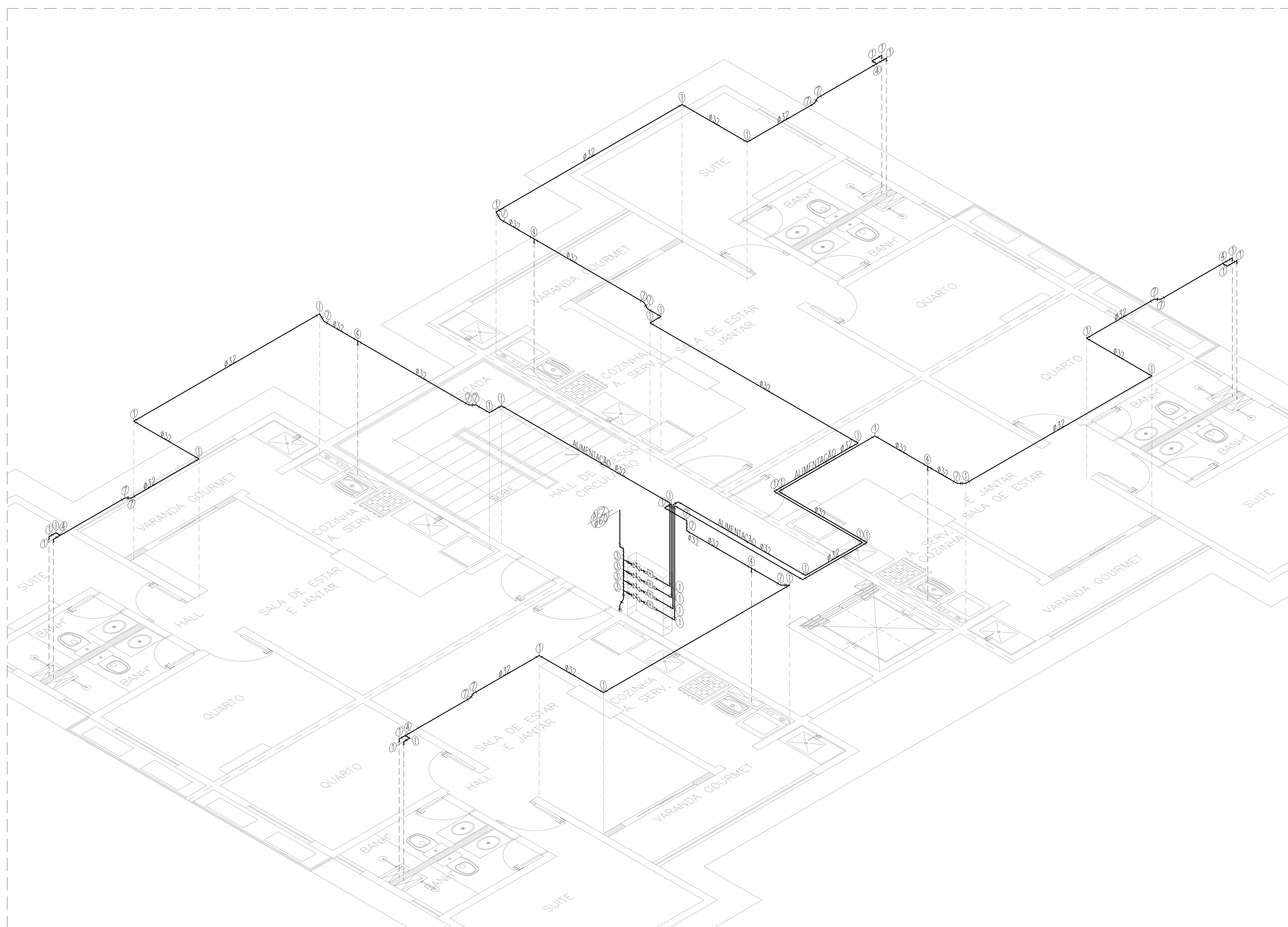
ISOMÉTRICO BLOCO TIPO B – 1º PAVIMENTO. ESC. 1/35
