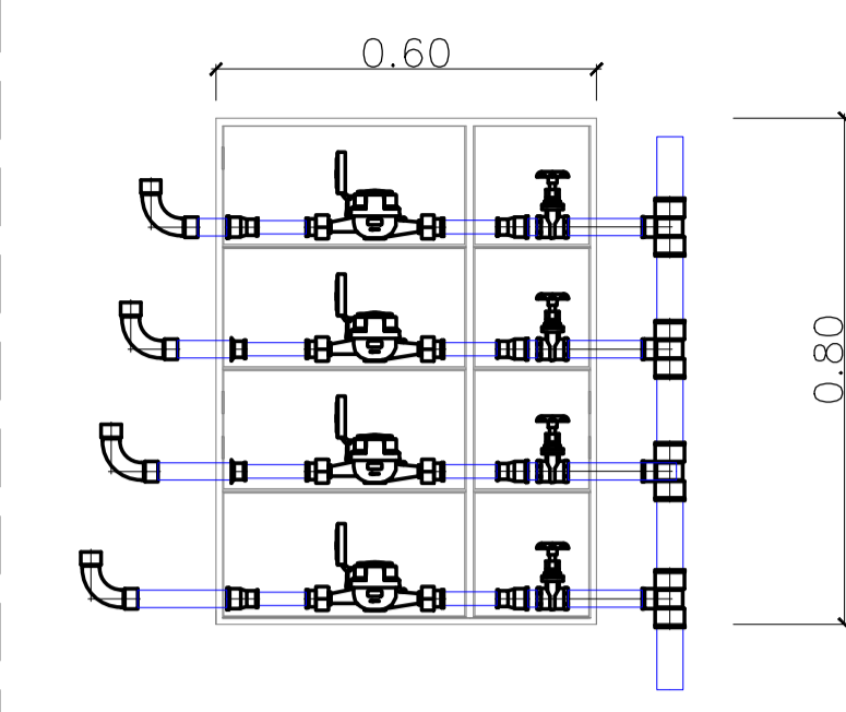
DETALHE – CAIXA DE HIDRÔMETRO SEM /ESC.
