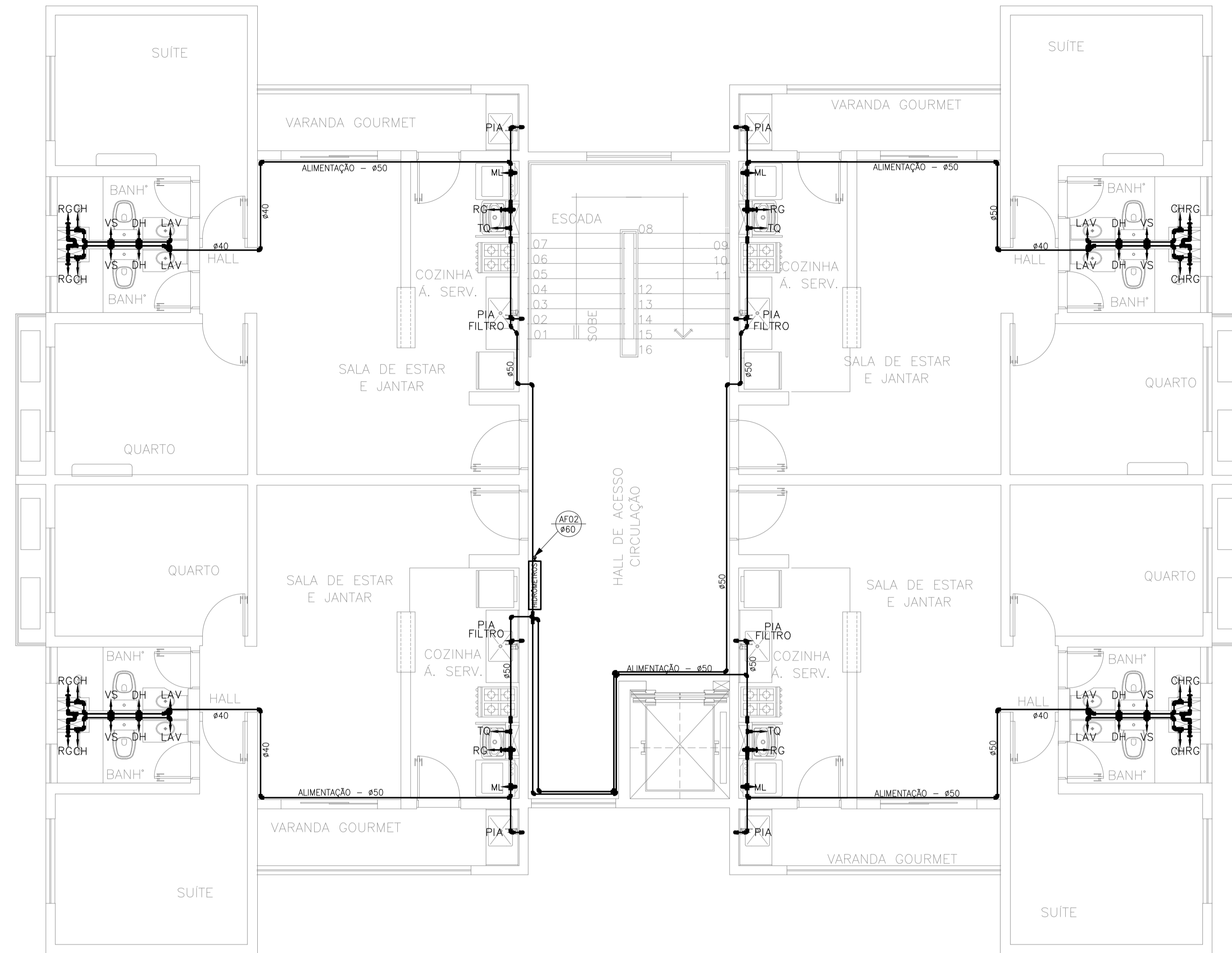
PLANTA BAIXA – PAV. TIPO/3º PAVIMENTO – BLOCO TIPO B ESC. 1/50
