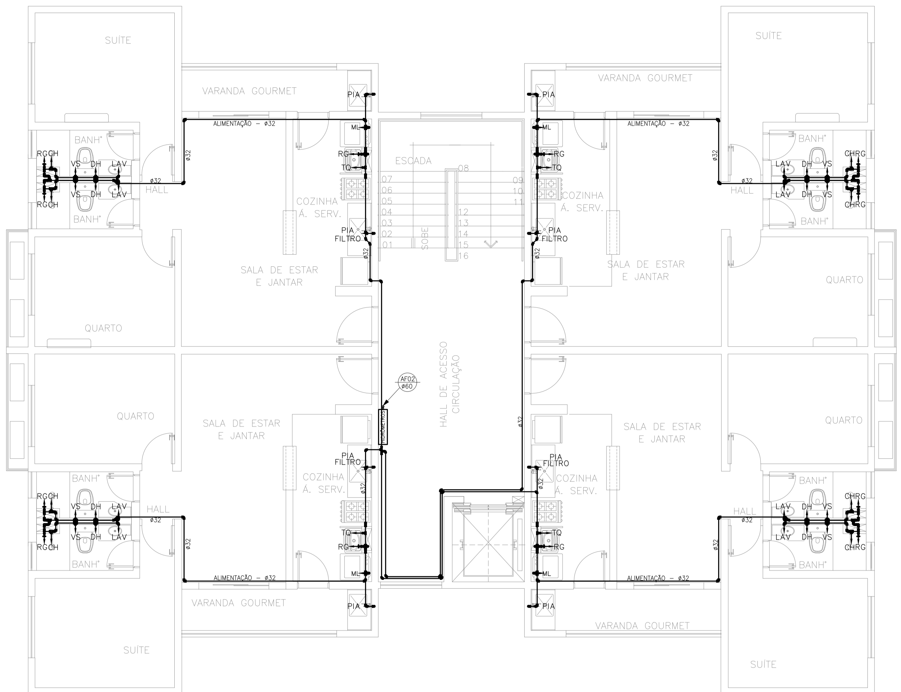
PLANTA BAIXA – PAV. TIPO/1º E 2º PAVIMENTO – BLOCO TIPO B ESC. 1/50
