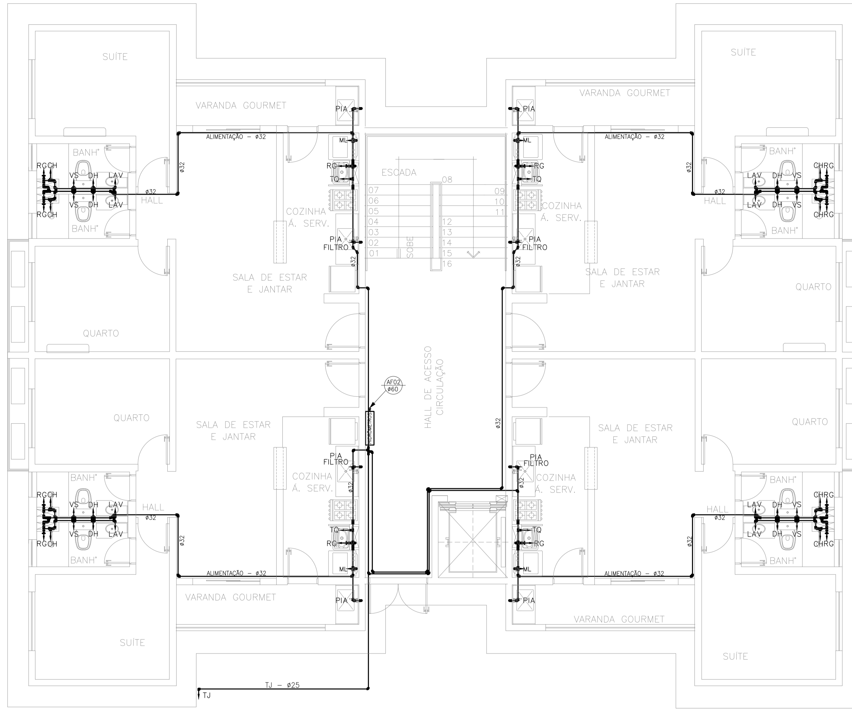
PLANTA BAIXA – PAV. TÉRREO – BLOCO TIPO B ESC. 1/50
