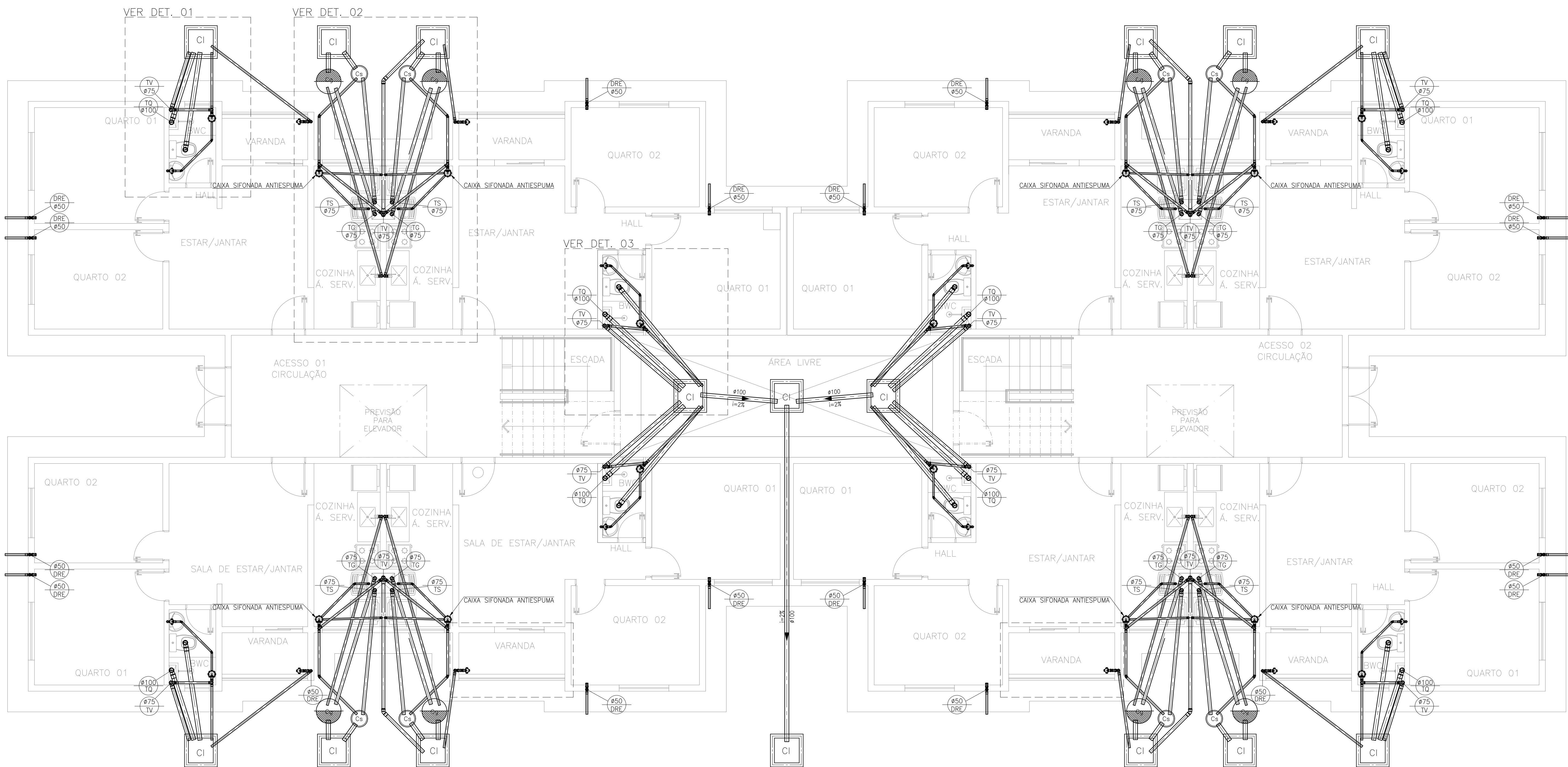
PLANTA BAIXA — PAV. TÉRREO BLOCO TIPO 2 — 32 APTO ESC. 1/50
