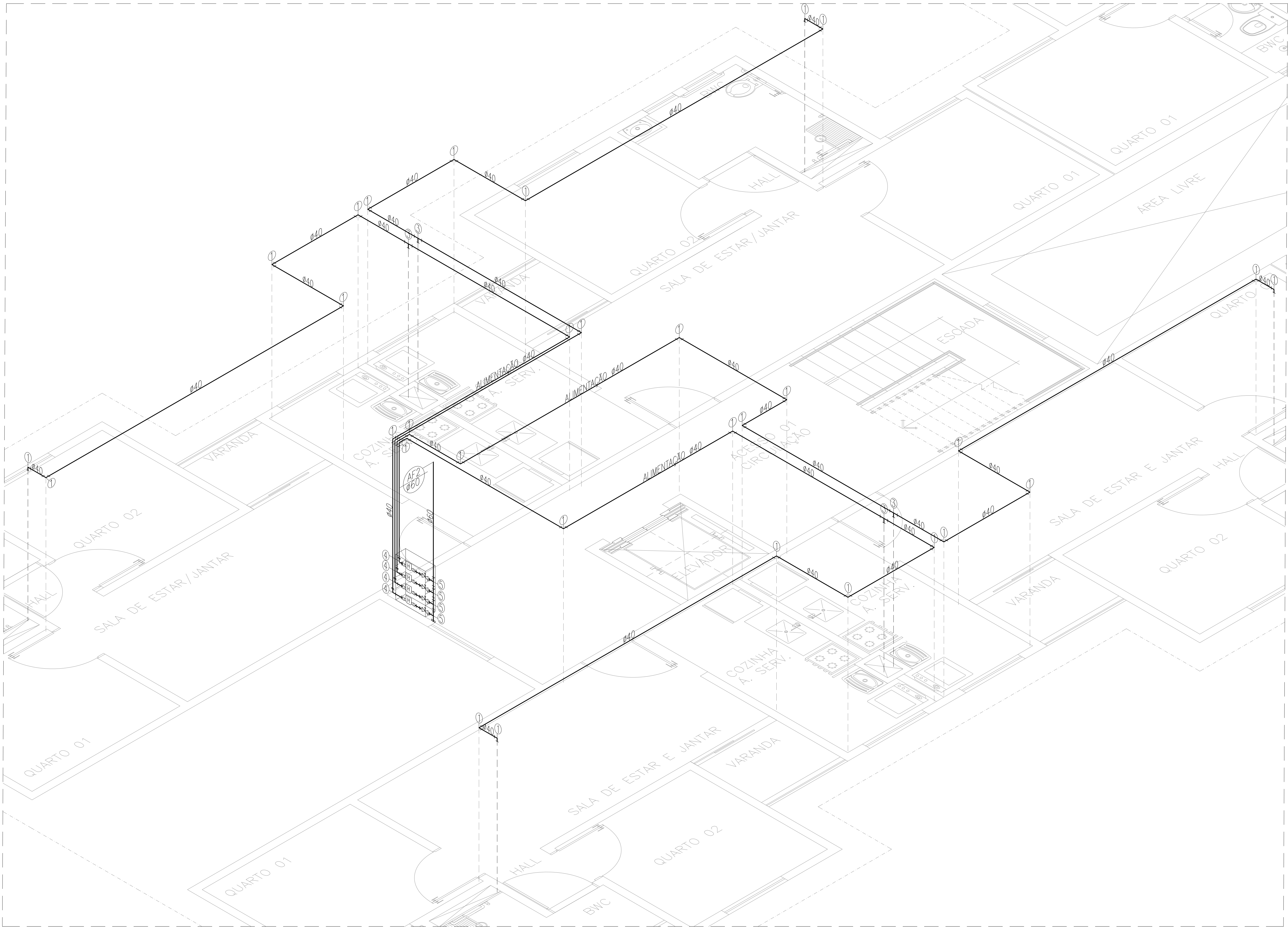
ISOMÉTRICO – 3º PAVIMENTO. ESC. 1/30
