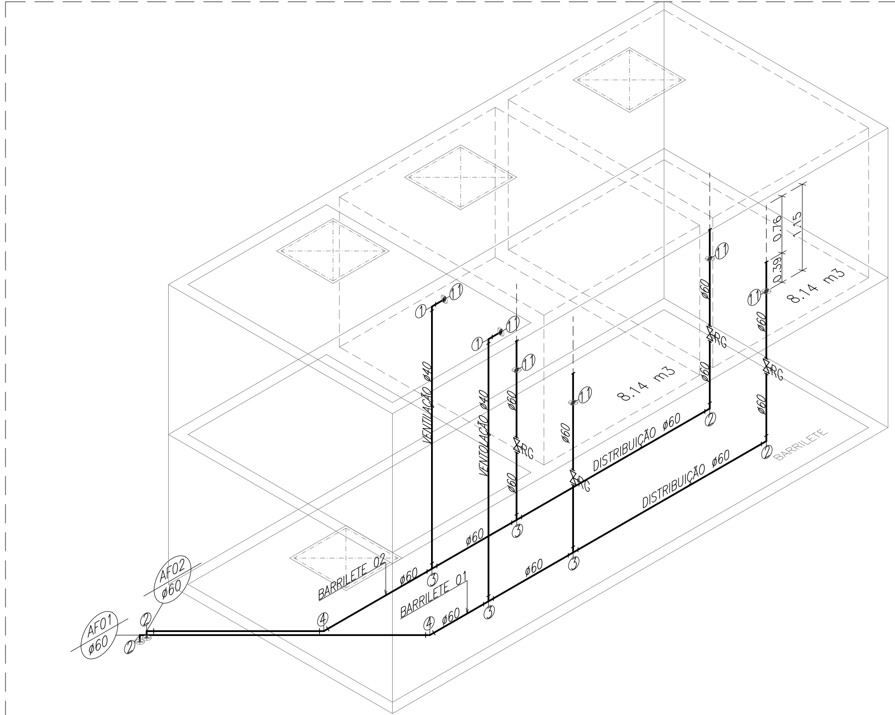
DETALHE ISOMÉTRICO CAIXA D'ÁGUA – DISTRIBUIÇÃO
