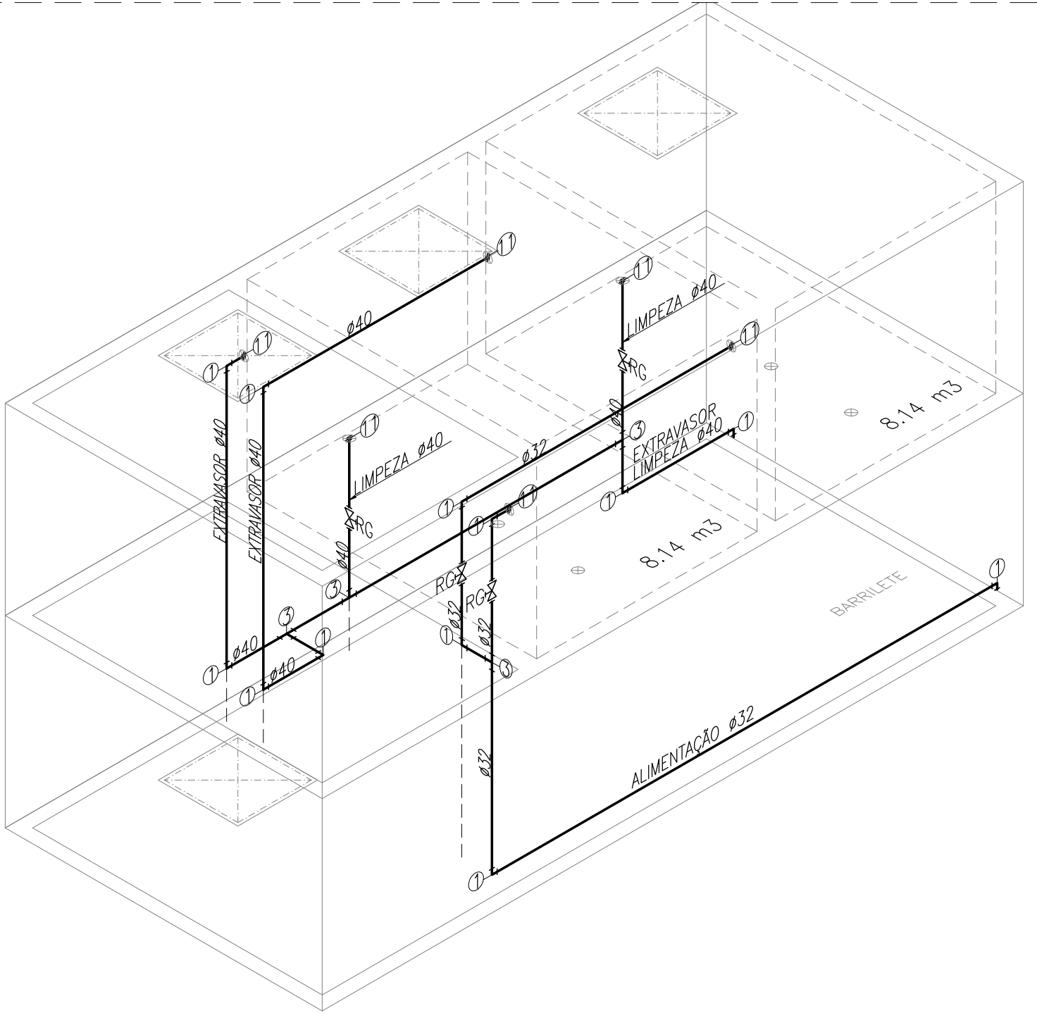
DETALHE ISOMÉTRICO CAIXA D'ÁGUA – ALIMENTAÇÃO EXTRAVASOR/LIMPEZA ESC. 1/50
