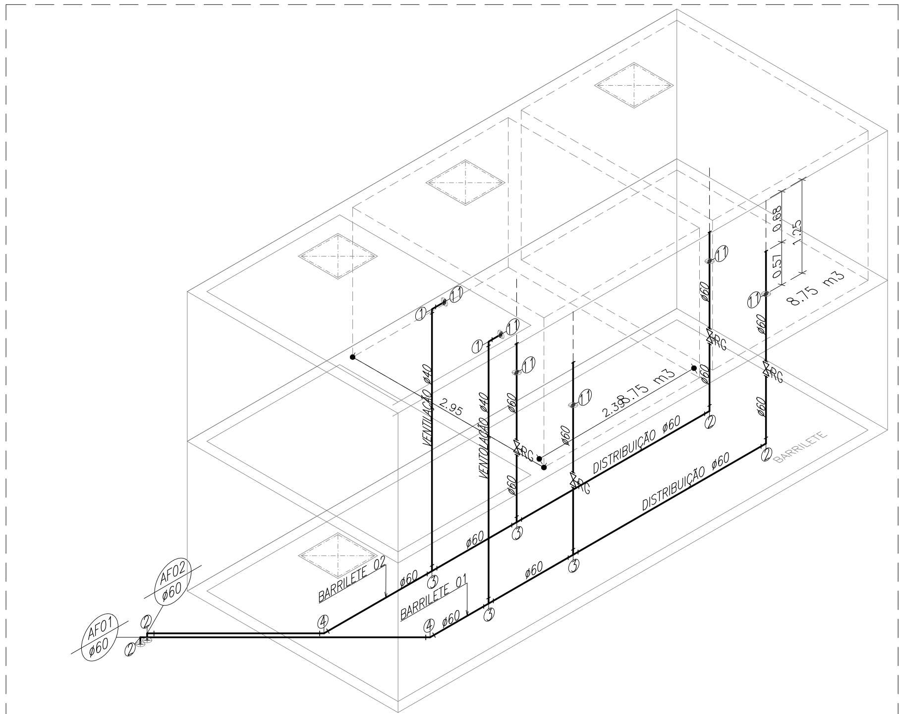
DETALHE ISOMÉTRICO CAIXA D'ÁGUA — DISTRIBUIÇÃO BARRILETE 01 E 02 ESC. 1/50
