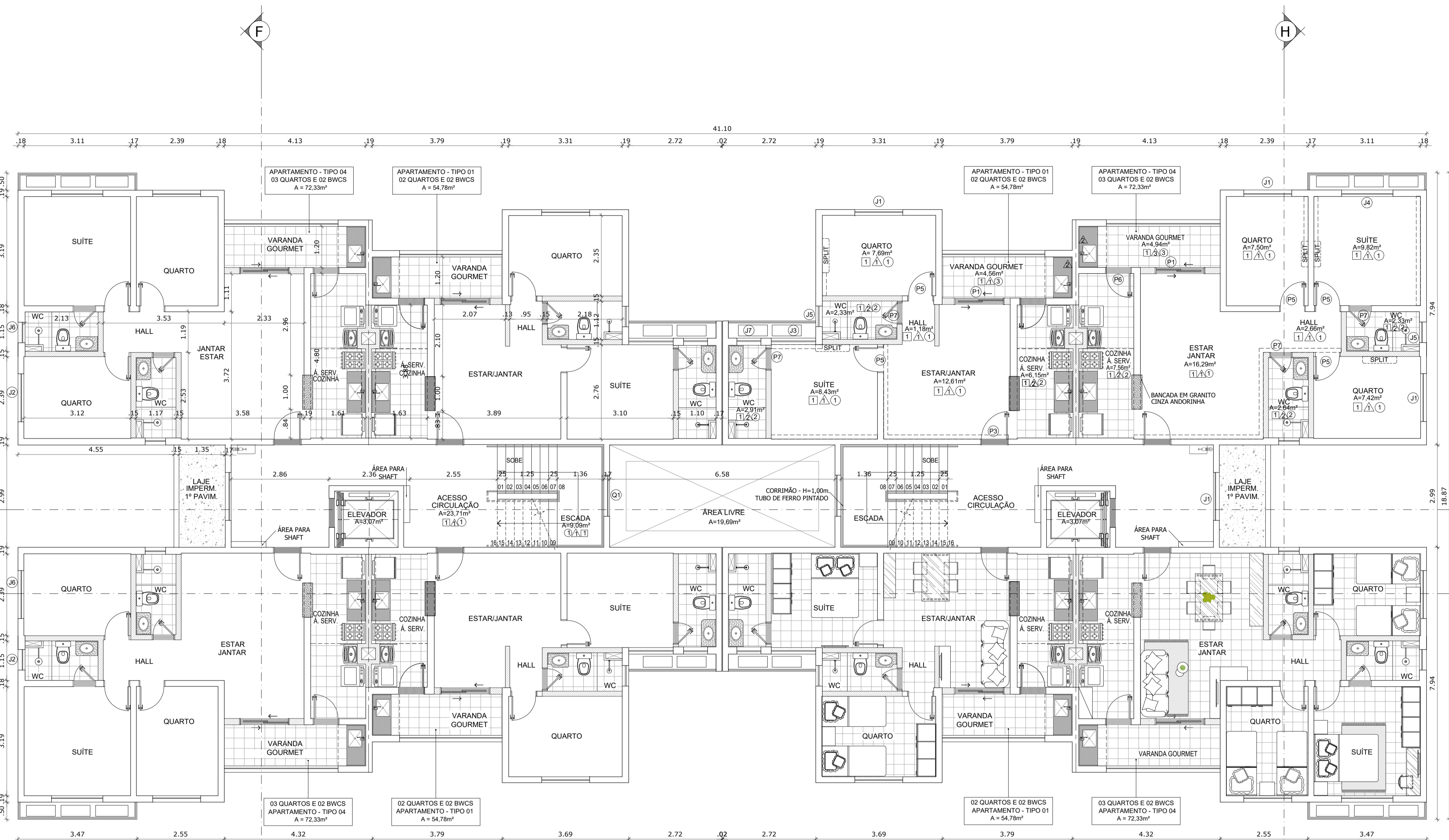
PLANTA BAIXA - PAVIMENTO TIPO CONDOMÍNIO JARDINS DO TURU 3 Escala: 1/75
