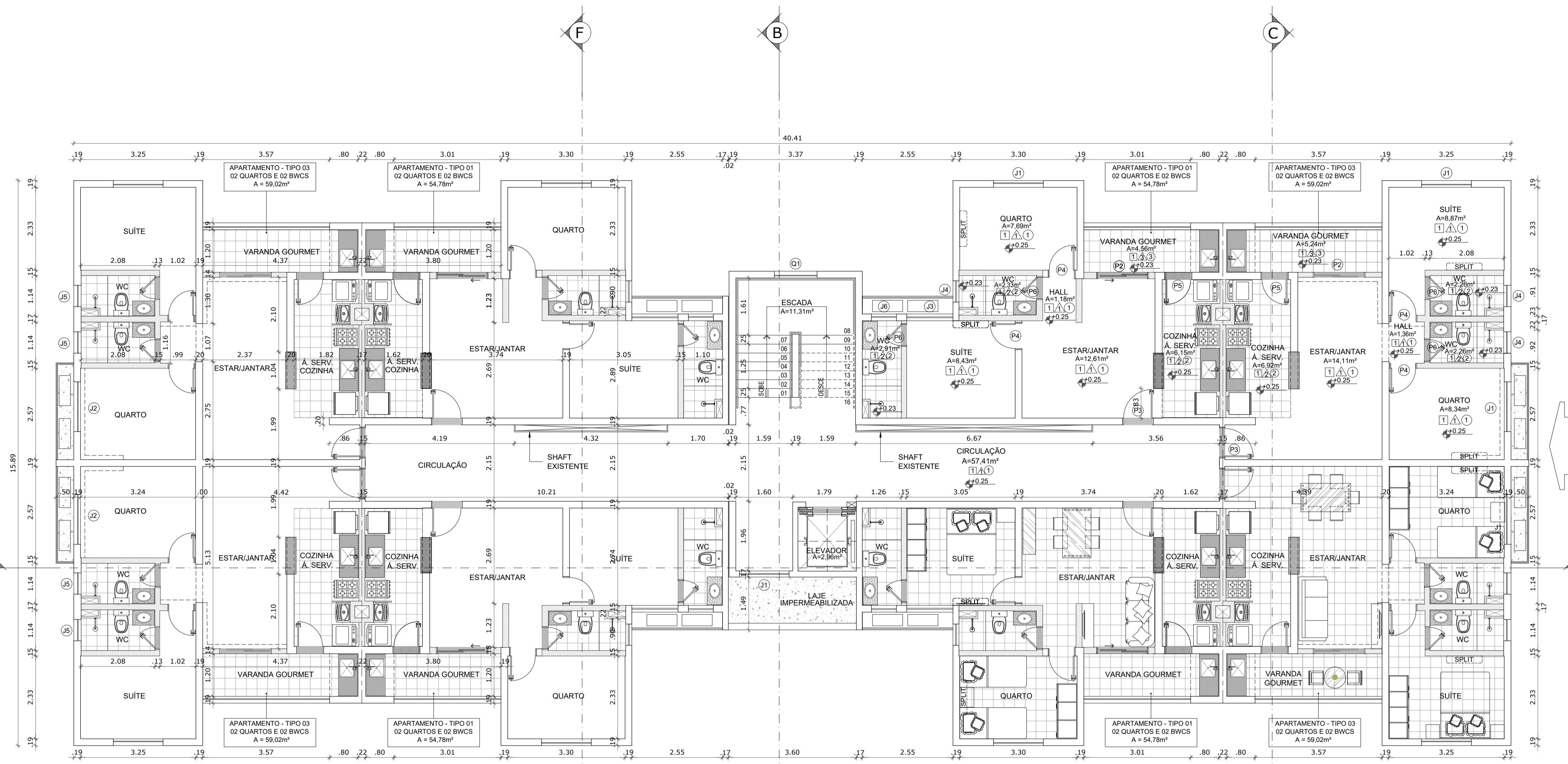
PLANTA BAIXA - PAV. TIPO CONDOMÍNIO JARDINS DO TURU 3 Escala: 1/75
